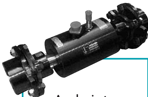
Acoplamiento transductor de par El acoplamiento espaciador especial tiene un transductor de par incorporado para utilizar en aparatos de pruebas. El dispositivo se utiliza para probar transmisiones de vehículos todo terreno.
