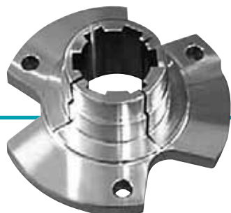
Núcleos ranurados estilo abrazadera Para embrague positivo alto. Elimina la necesidad de chavetas y reduce la vibración en aplicaciones de eje ranurado.
