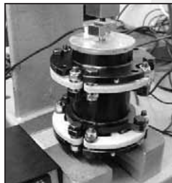
Prueba de resistencia axial del acoplamiento
