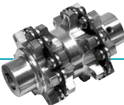
Acoplamientos de doce pernos Provee alta resistencia a la torsión y registro mejorado
